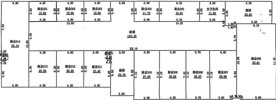
三层平面图，整层共 660.97m 2 （14 间）
