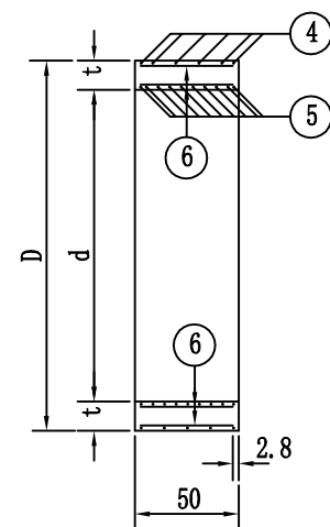
0.5米正管节纵断面
