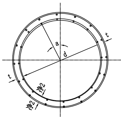
管节横断面
