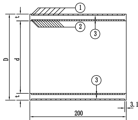
2米正管节纵断面
