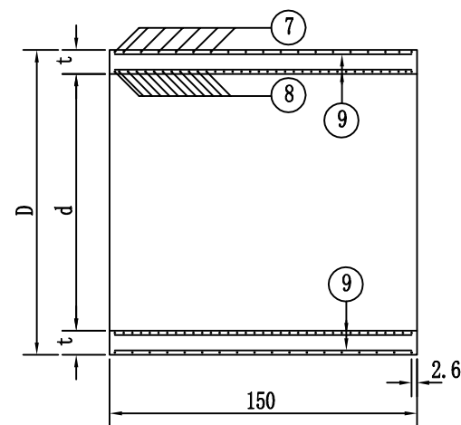
1.5米正管节纵断面
